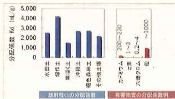
図 1 国内土壌の放射性 Cs と有害物質の分配係数
