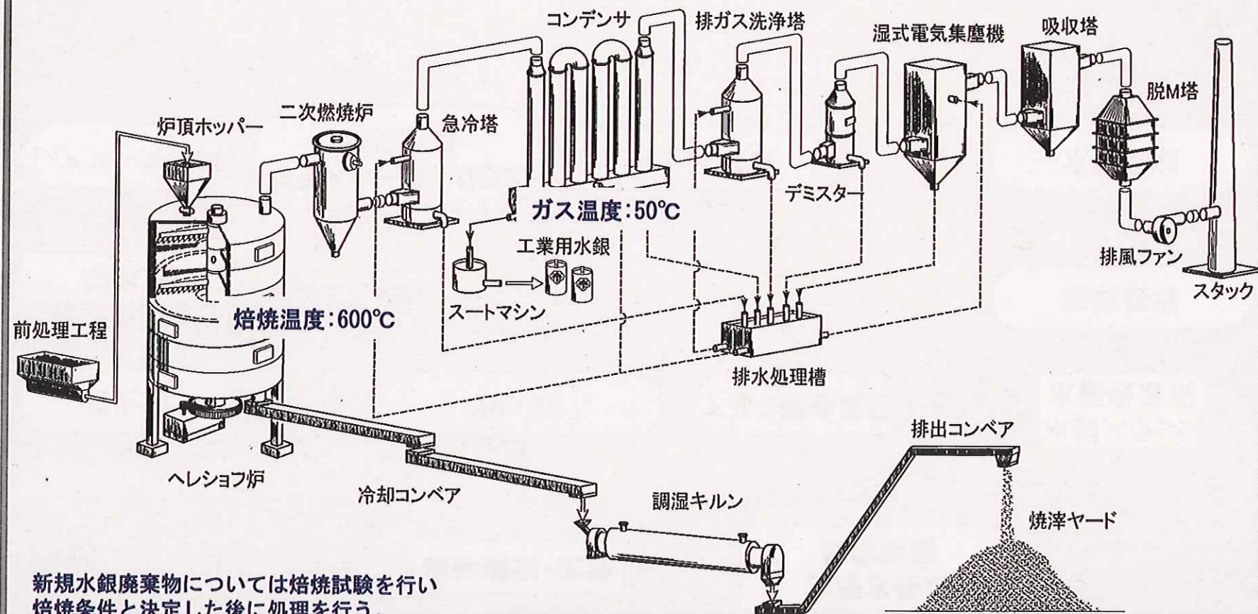
ヘレショフ炉処理工程図
