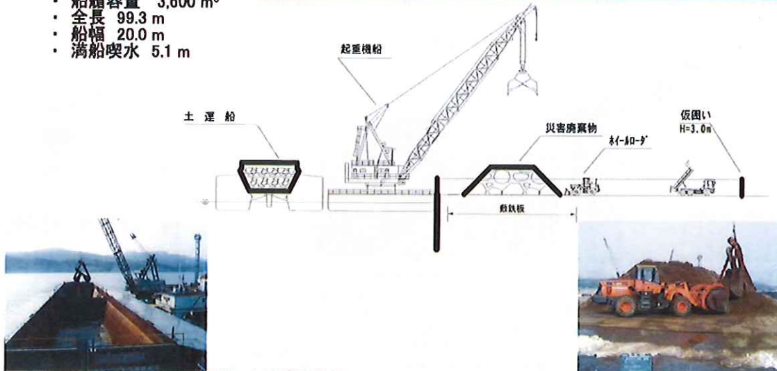
ホイールローダによる補助状況
