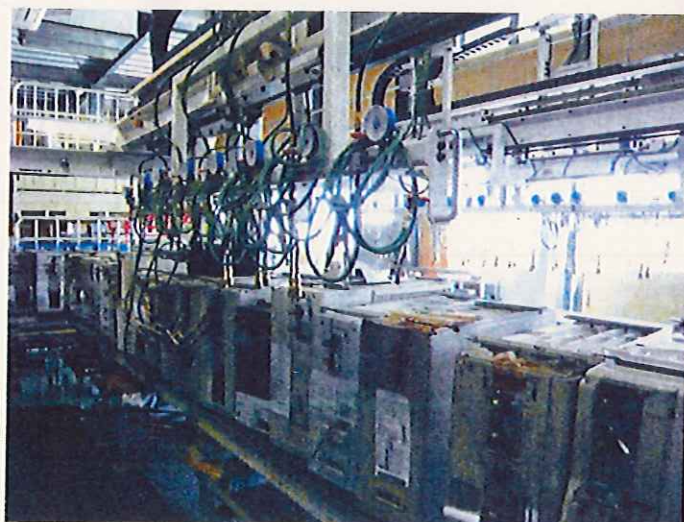
エアコンの冷媒フロン回収ライン
